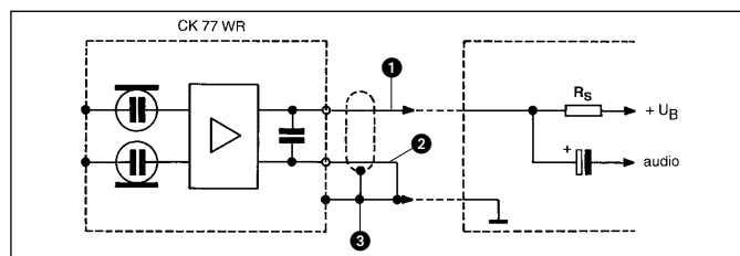
Fig. 2: Diagrama de circuitos del CK 77 WR
