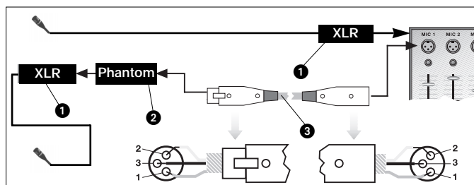
Fig. 3: Conexión a una entrada balanceada
