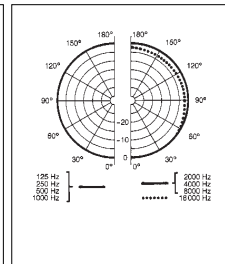
Polardiagramm
