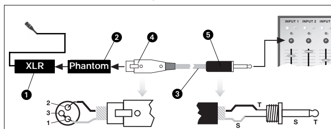
Fig. 4 : Raccordement sur une entrée asymétrique
