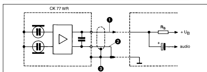
Fig. 2: Esquema elétrico do CK 77 WR
