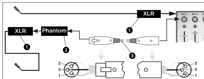
Fig. 3: Conexão a uma entrada balanceada
