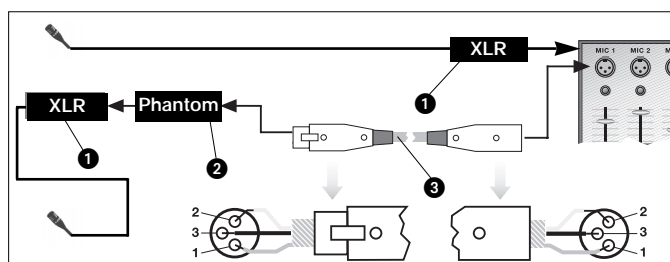
Fig. 3 : Raccordement sur une entrée symétrique
