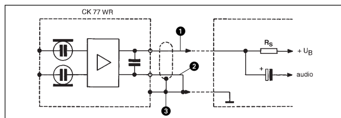
Abb. 2: Schaltplan des CK 77 WR
